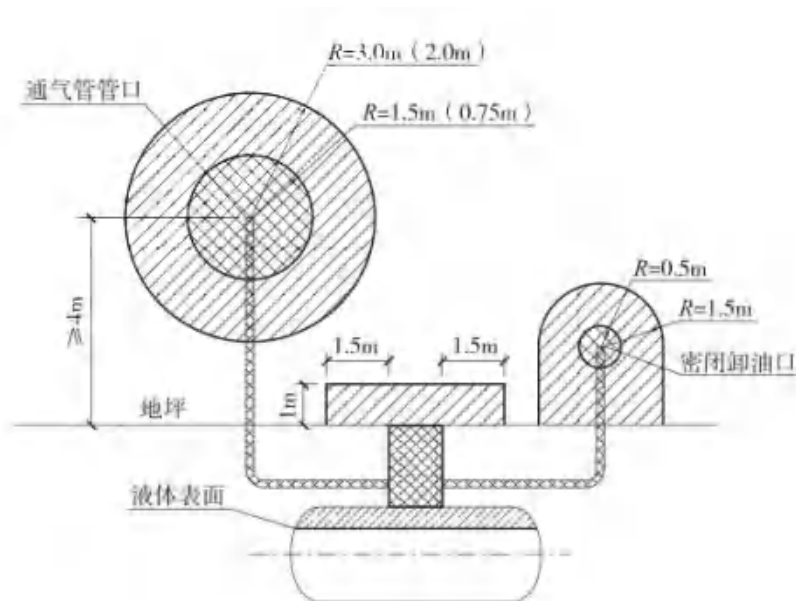
图 3.4-3 埋地卧式汽油储罐爆炸危险区域划分
