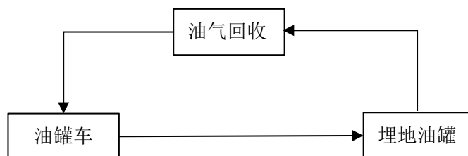
图 2.4-1 汽油卸油工艺流程图
