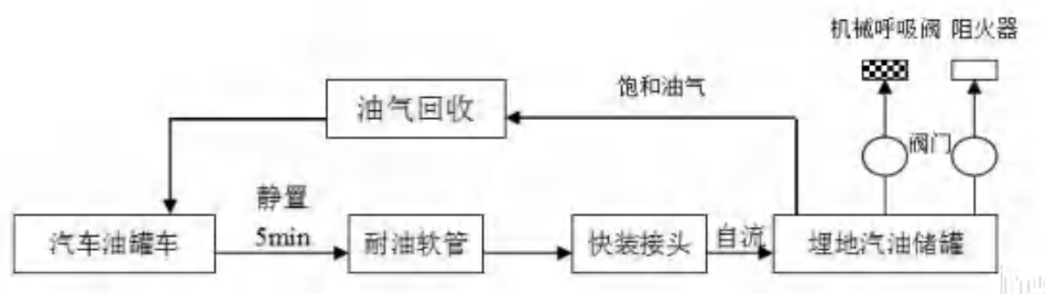
图 2.3-1 加油站汽油卸油工艺流程图
