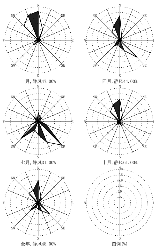
图 2.2.3 加油站所在区域的风向频率玫瑰图
