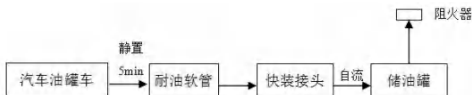
图 2.3-2 柴油卸油工艺流程图
