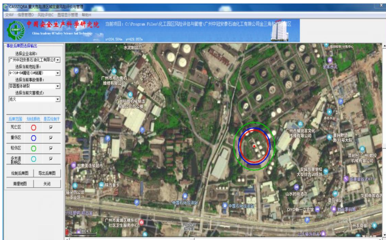
图 7.2-12 1#储罐（1000 立方米）容器整体破裂事故后果图
