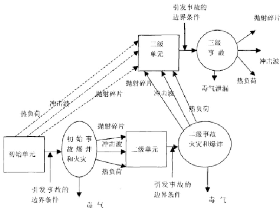
图 7.5-1 多米诺效应模型
