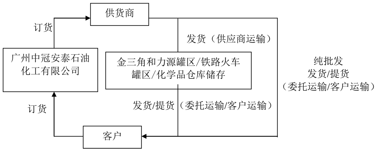
图 2.8-1 危险化学品经营活动流程图
