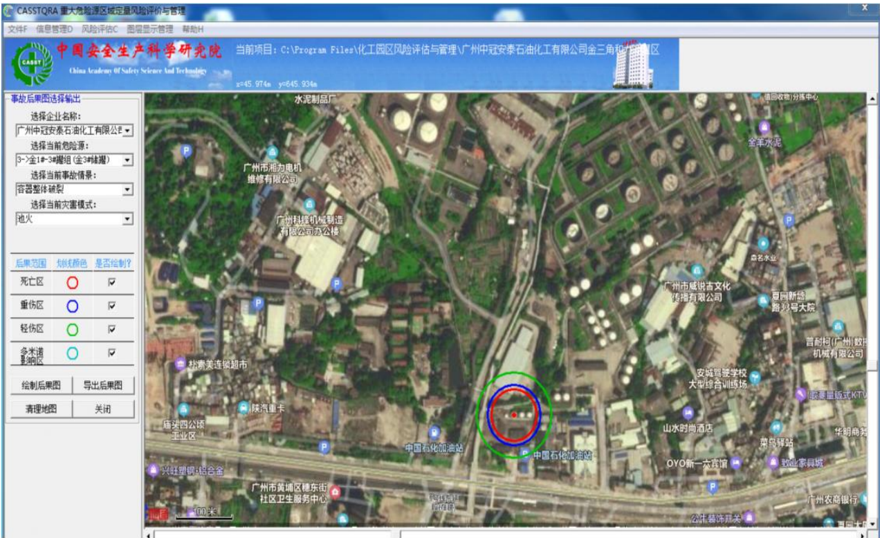
图 7.2-11 金 3#储罐（300 立方米）容器整体破裂事故后果图
