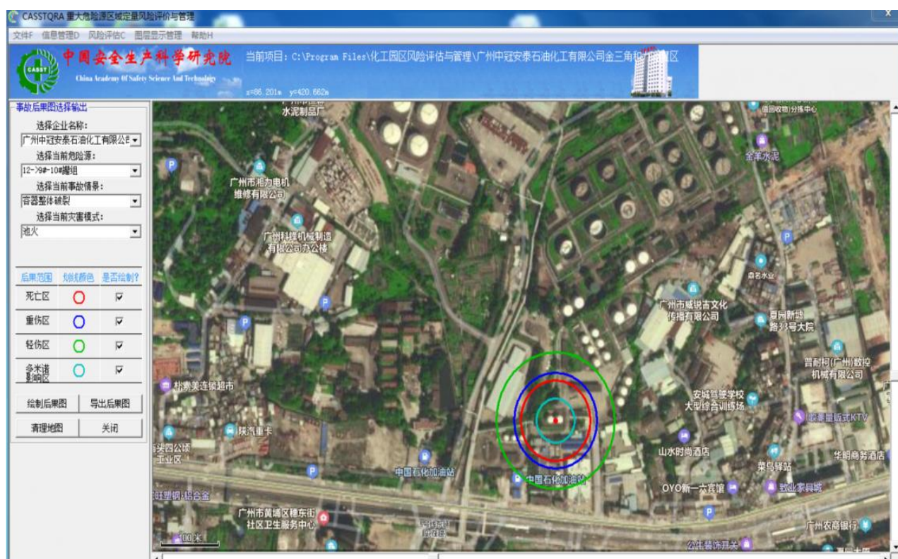
图 7.2-13 9#~10#罐组（2×1000 立方米）容器整体破裂事故后果图
