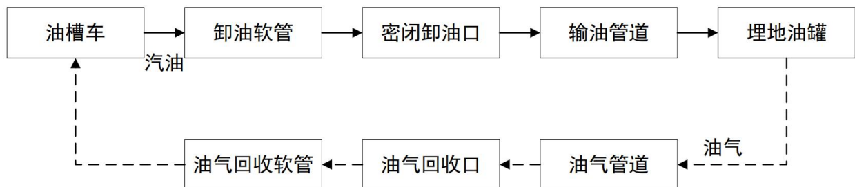
图 2.4-1 汽油卸油工艺流程
