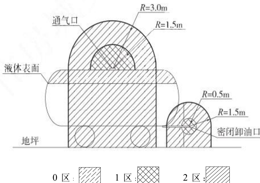
图 3.4-2 汽油油罐车和密闭卸油口的爆炸危险区域划分
