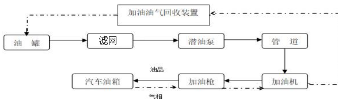
图 2.4-5 汽油加油工艺及加油油气回收工艺流程图
