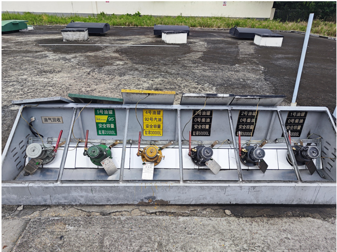
卸油口照片
