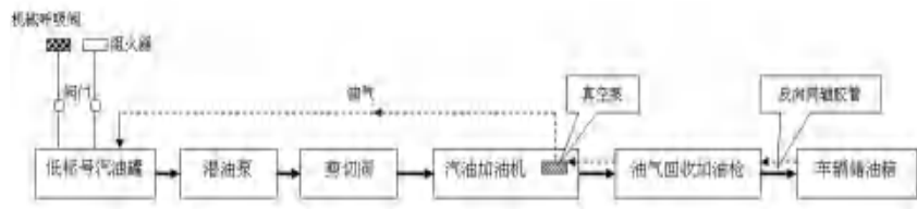
图 2.3-3 汽油加油工艺流程图
