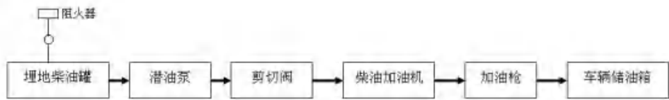
图 2.3-4 柴油加油工艺流程图
