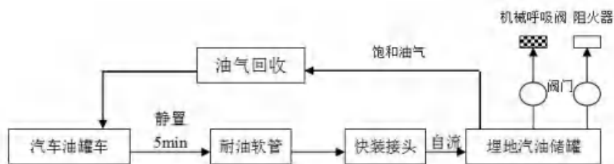
图 2.3-1 加油站汽油卸油工艺流程图
