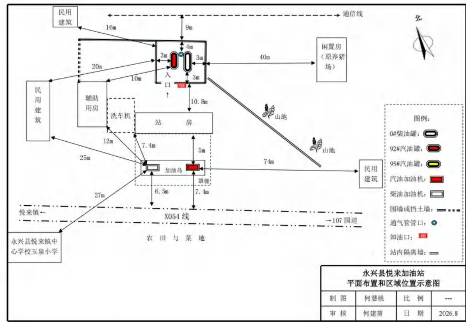
附图：加油站总平面布置和四至距离示意图
